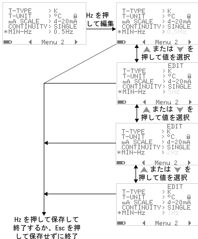
図 4-11 最小周波数のセットアップ
