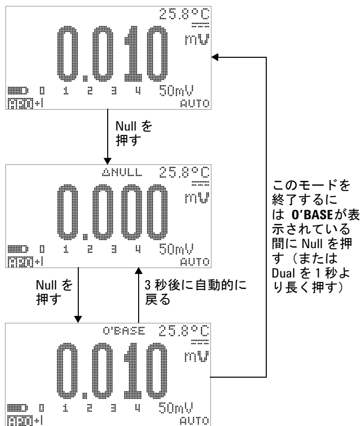
図 3-4 ノル (相対) モードの操作
