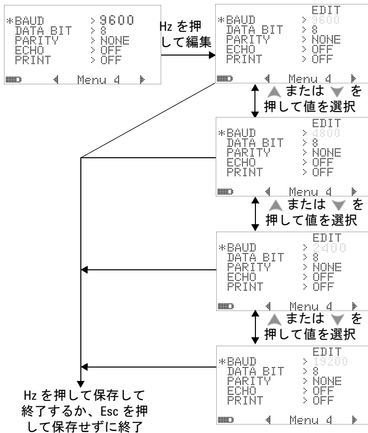
図 4-17 リモート制御のボーレートのセットアップ
