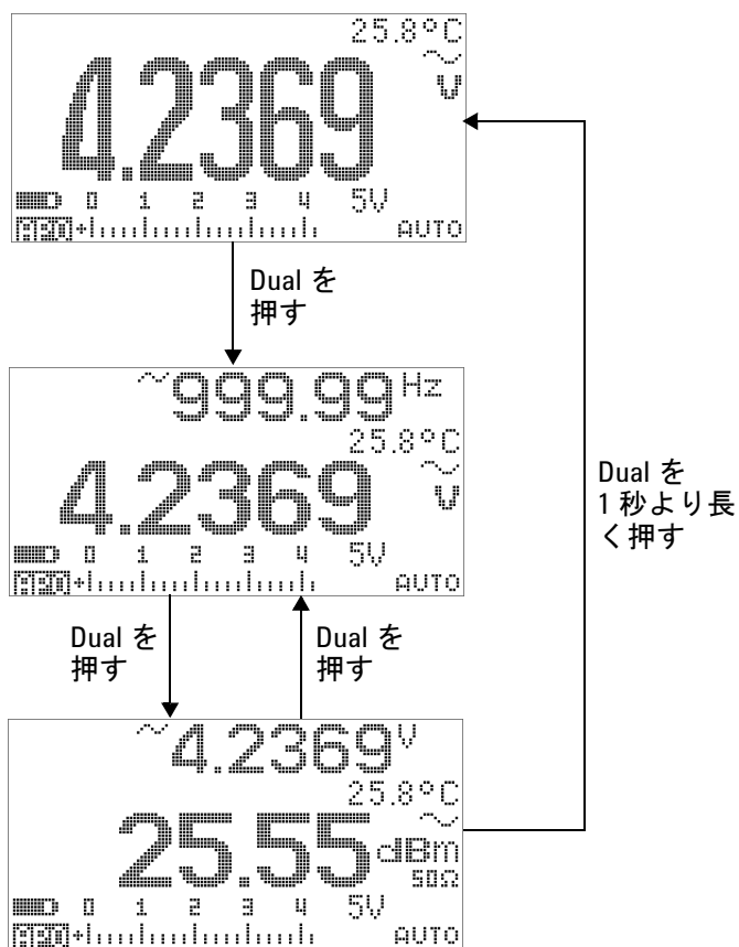
図 3-5 dBm 表示モードの操作
