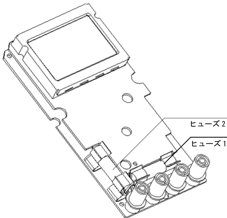
図 5-9 ヒューズの交換
