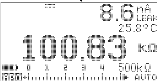
図 2-7 スマートΩをオンにしたときの表示のタイプ
