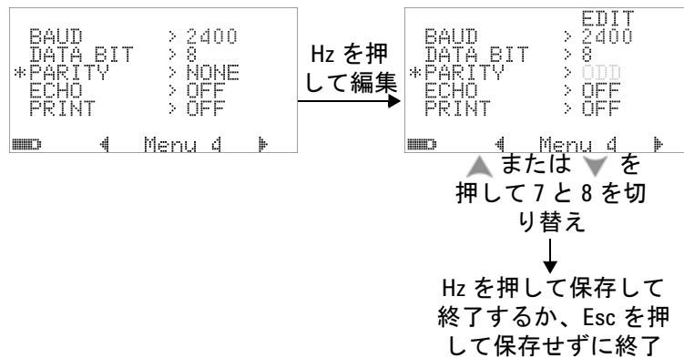
図 4-18 リモート制御のデータ・ビットのセットアップ
