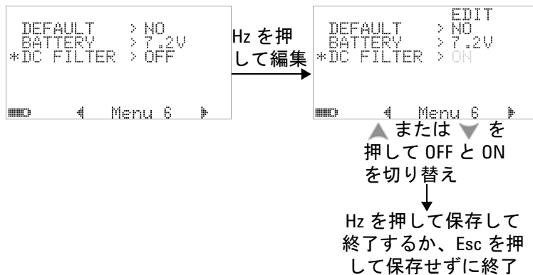
図 4-32 DC フィルタ
