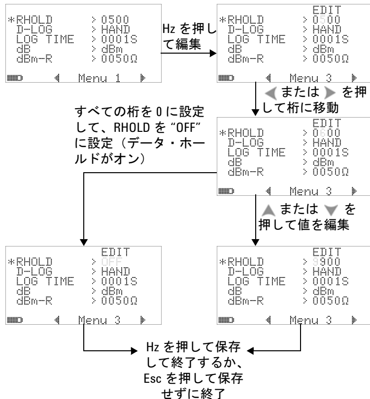
図 4-2 データ・ホールド／リフレッシュ・ホールドのセットアップ
