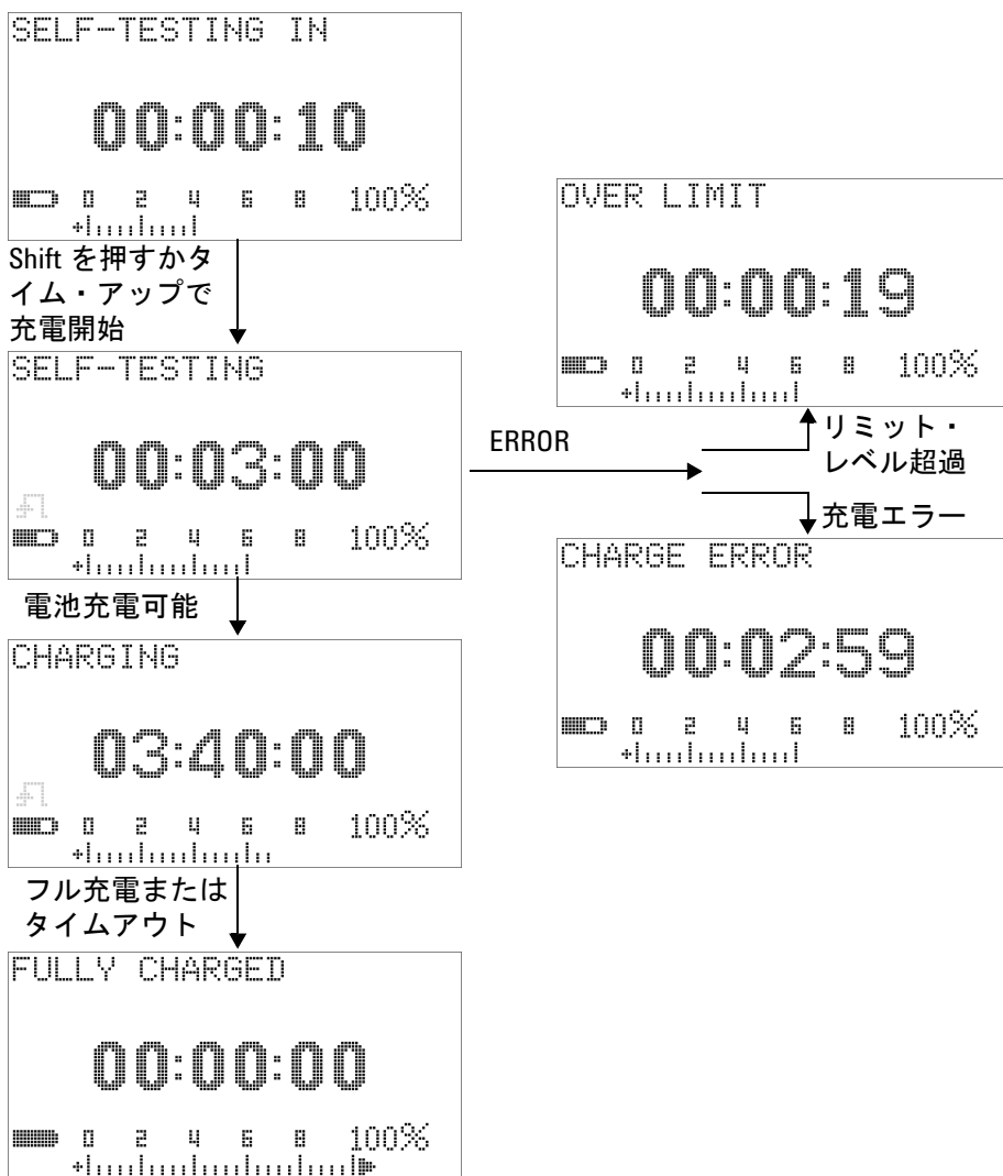
図 5-7 電池充電手順
