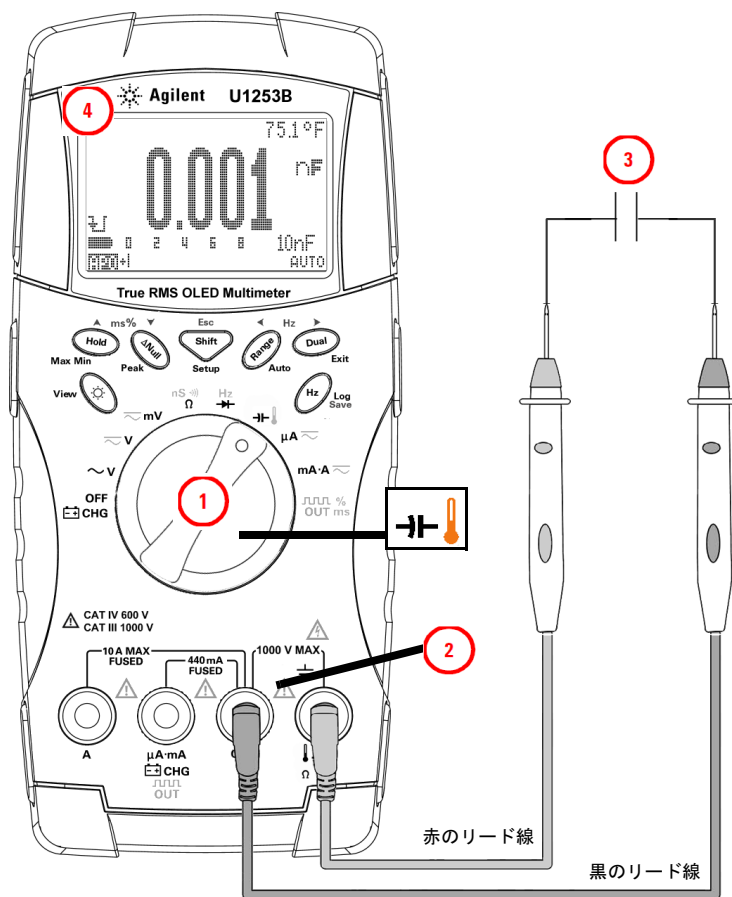
図 2-14 キャパシタンス測定
