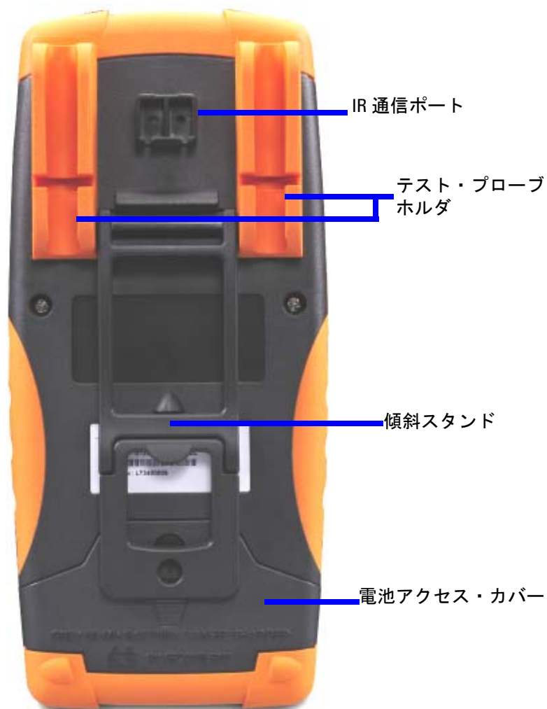
図 1-5 リア・パネル
