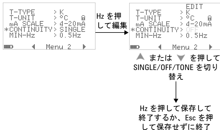
図 4-10 導通テストに使用するサウンドの選択
