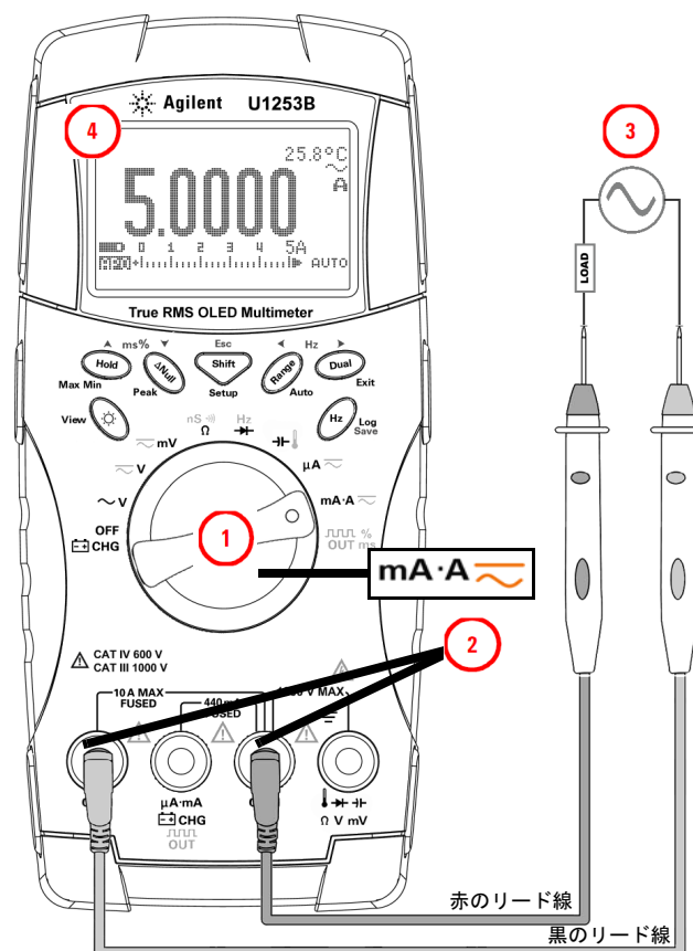
図 2-5 A (アンペア) 電流測定
