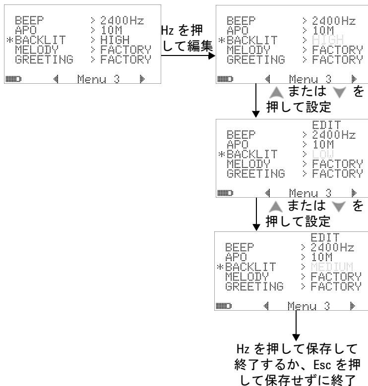
図 4-14 電源投入時バックライトのセットアップ
