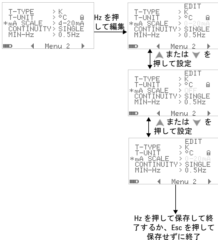
図 4-9 スケール表示値のセットアップ
