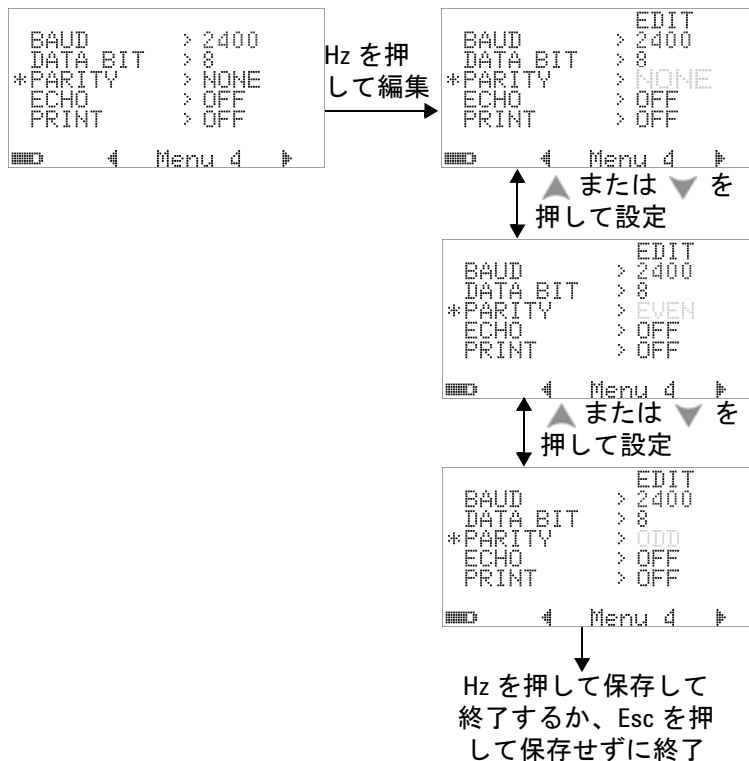
図 4-19 リモート制御のパリティ・チェックのセットアップ
