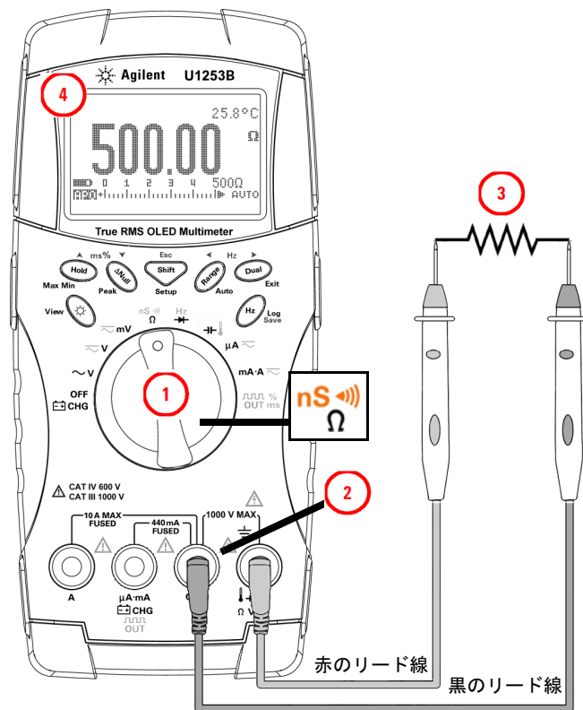
図 2-8 抵抗の測定
