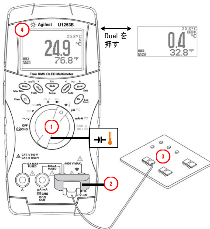
図 2-17 表面温度測定
