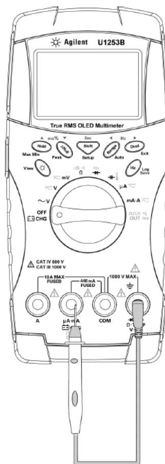
図 5-8 ヒューズのチェック手順
