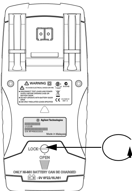
図 5-2 Agilent U1253B 真の実効値 OLED マルチメータのリア・パネル
