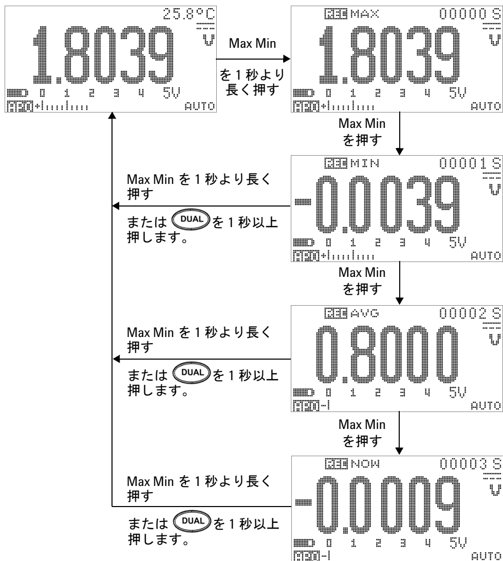
図 3-1 ダイナミック・レコーディング・モードの操作
